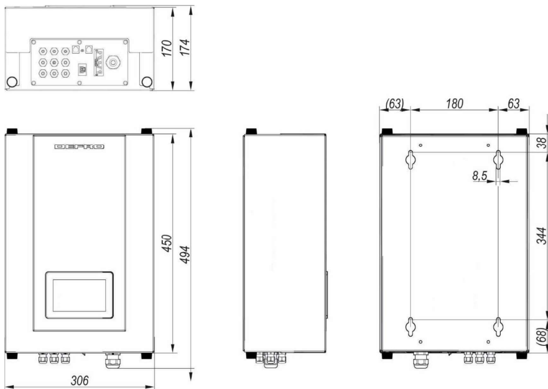
Rysunek 10. Wymiary skrzynki instalacyjnej DS: pompy ciepła DHPi MONOTEC.
