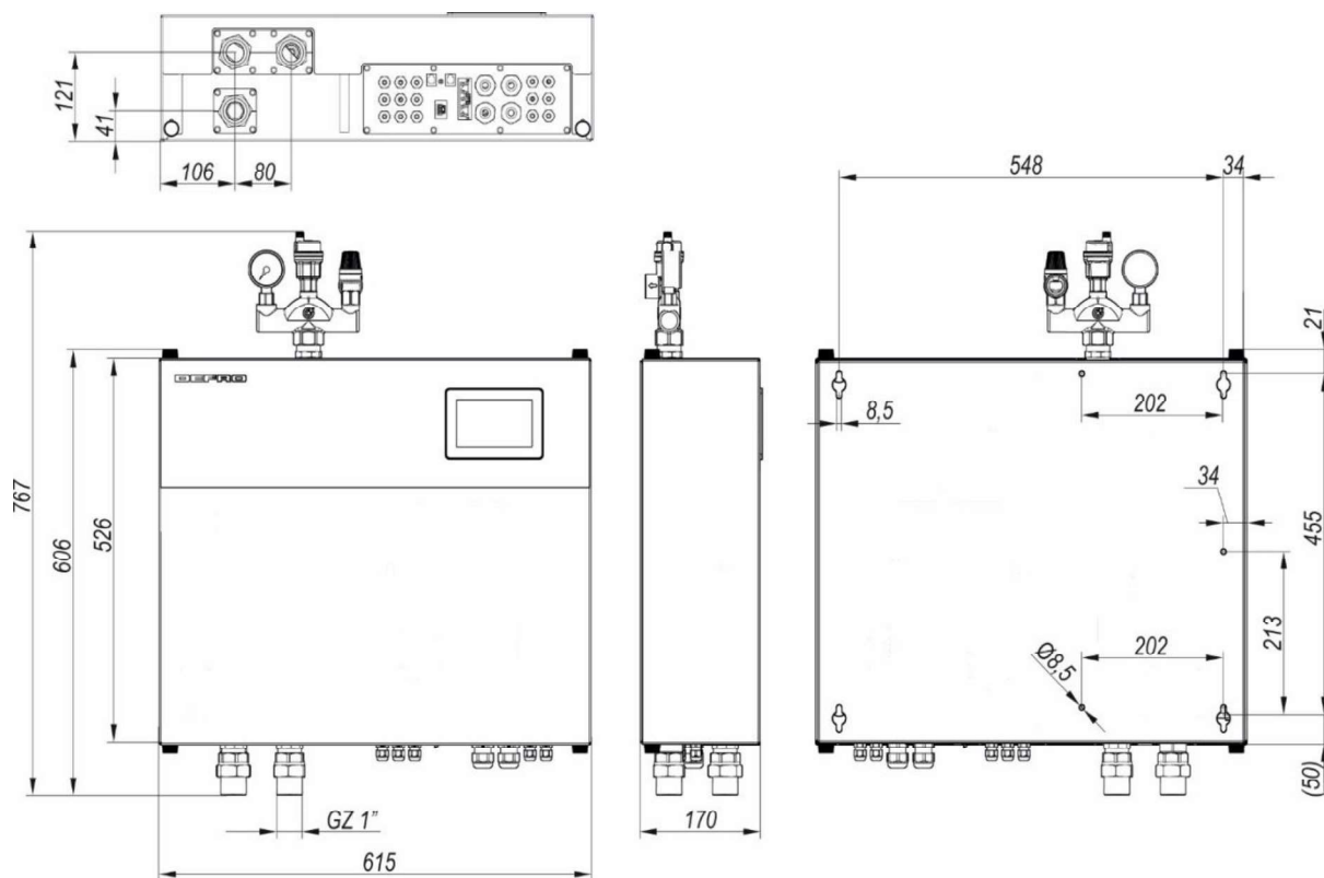
Rysunek 11. Wymiary hydromodułu DFi pompy ciepła DHPi MONOTEC.
