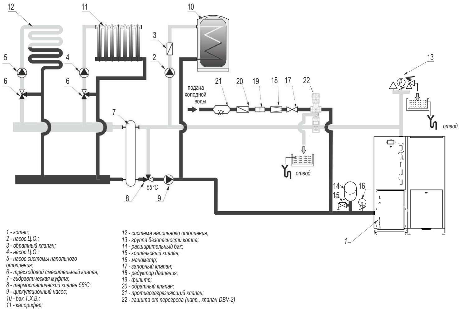
Изображение 10. Упрощенная схема системы отопления открытого типа
