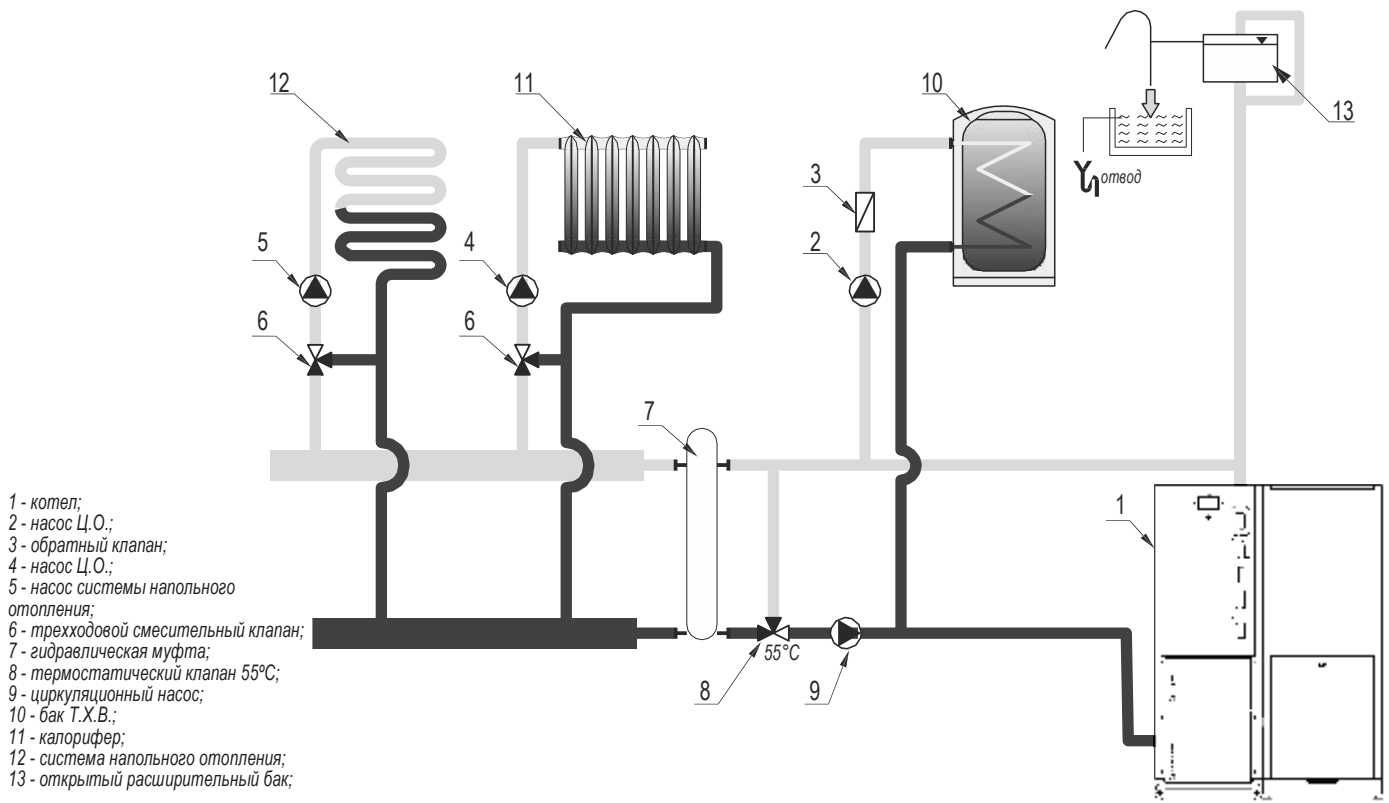
Изображение 10. Упрощенная схема системы отопления открытого типа
